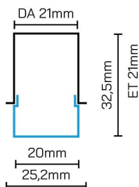
Abdeckung opal/hoch
